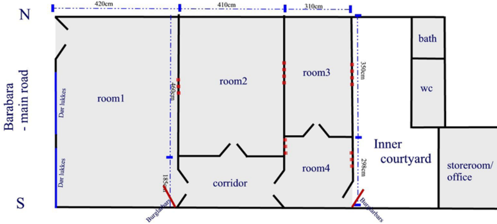
Grundplan
